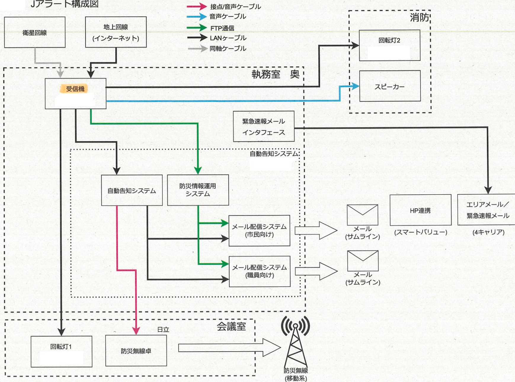
Jアラート構成図
