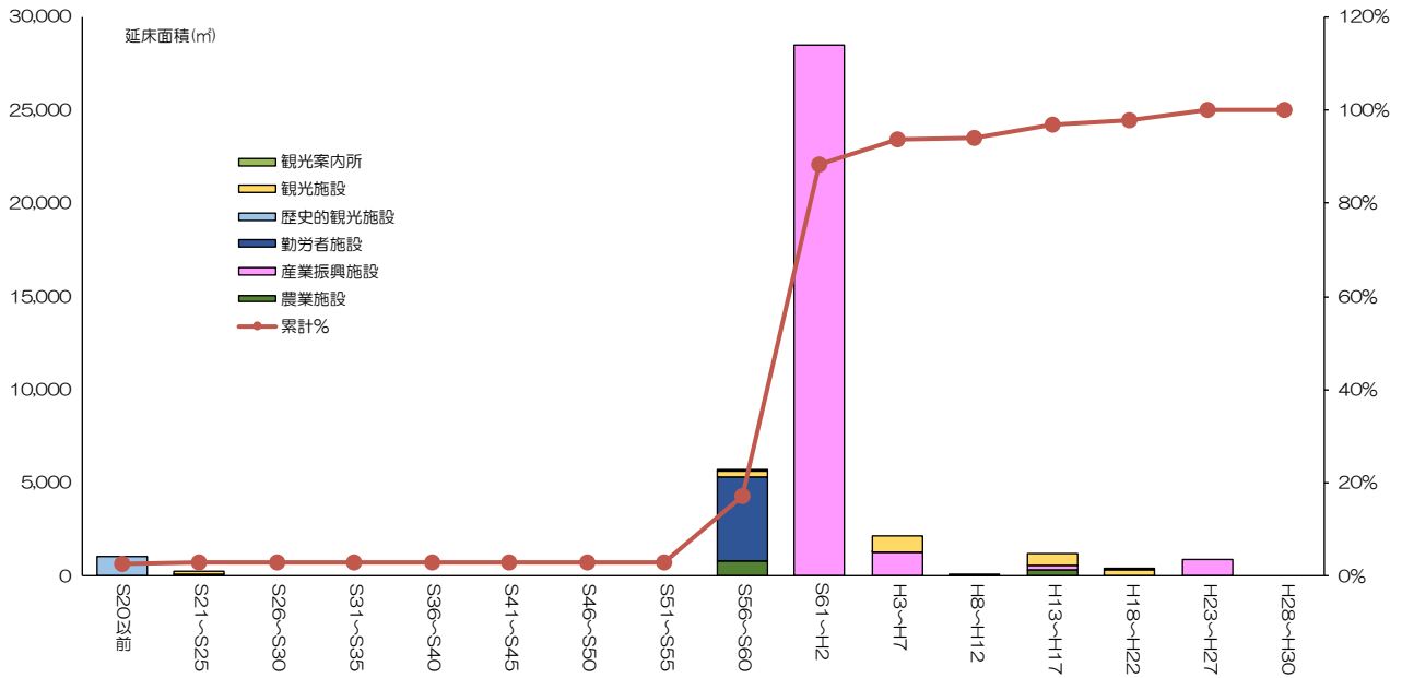
図 14-1 建築年度別の建物延床面積（産業・観光施設）
