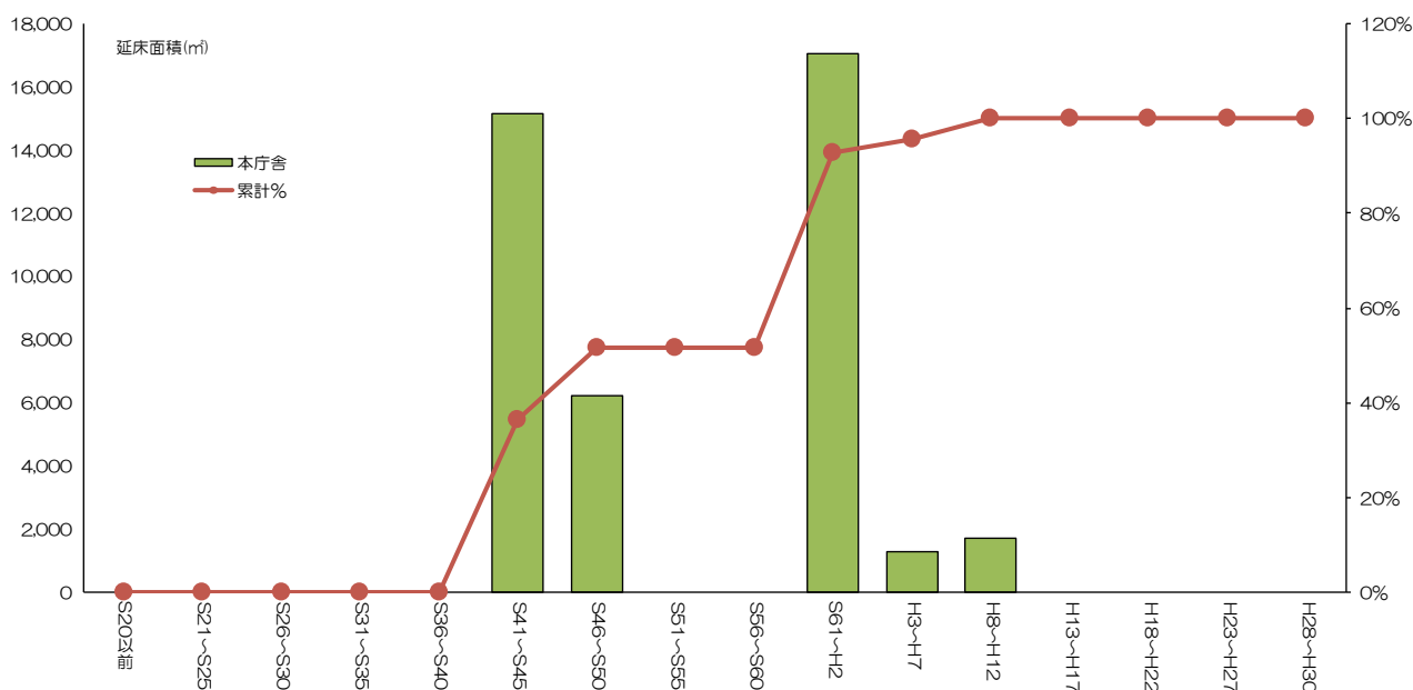
図 10-1 建築年度別の建物延床面積（本庁舎）
