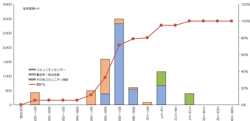
図 3-1 建築年度別の建物延床面積（コミュニティ施設）
