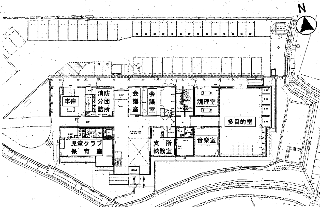
1階平面図
