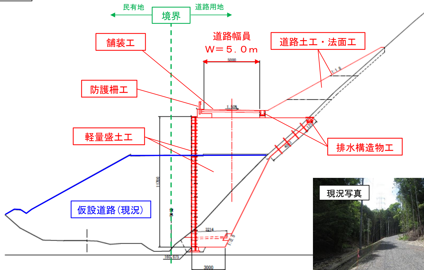
横断図
