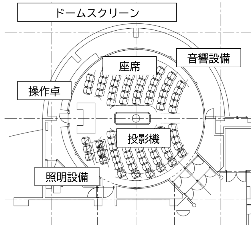
平面図(更新後)
