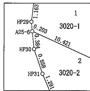
拡大図① S=1:50
