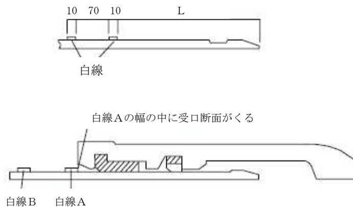
図 2.2.2.3-2 受口・挿し口の挿入完了（単位：mm）
