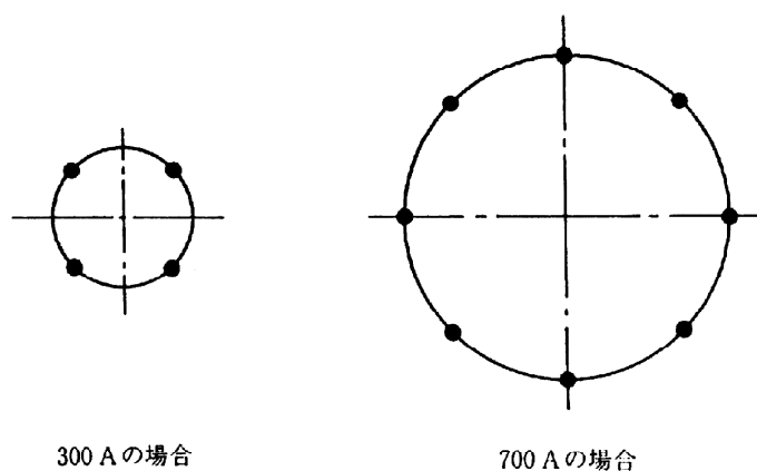
図 2. 2. 3. 6 仮付けの位置の例
