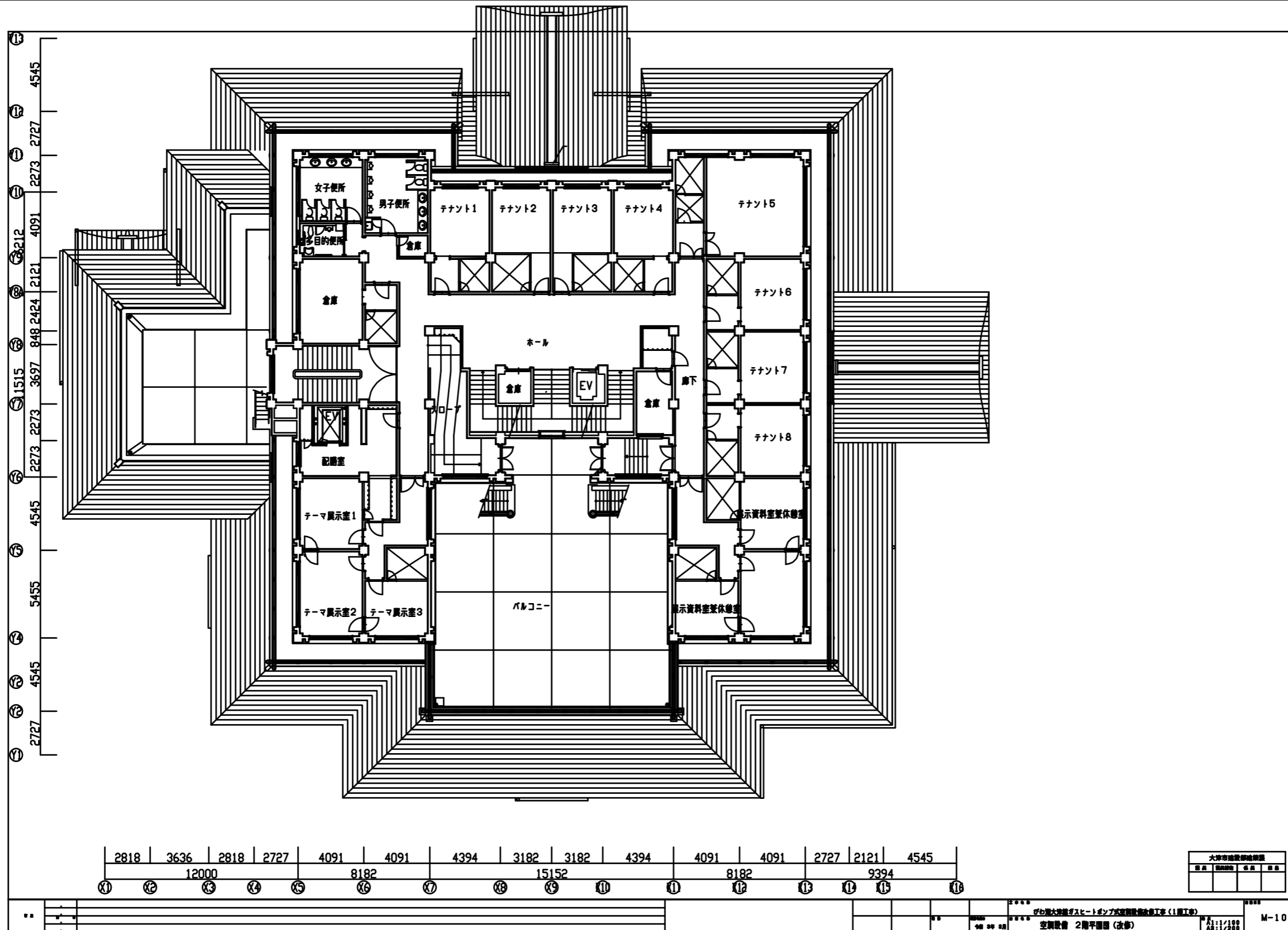
びわこ大津館 平面図 (2F)
