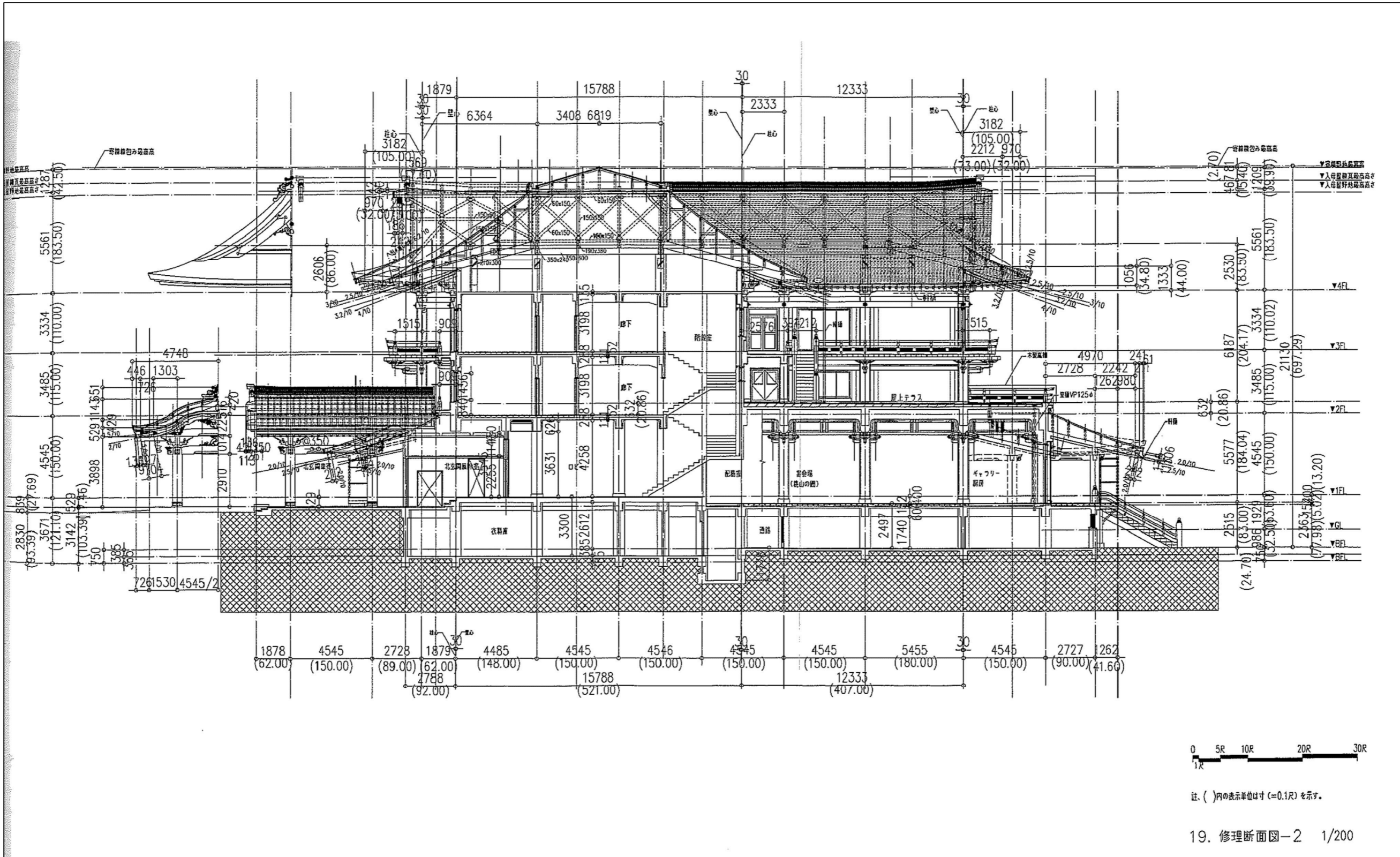
びわこ大津館 立面図 (2)
