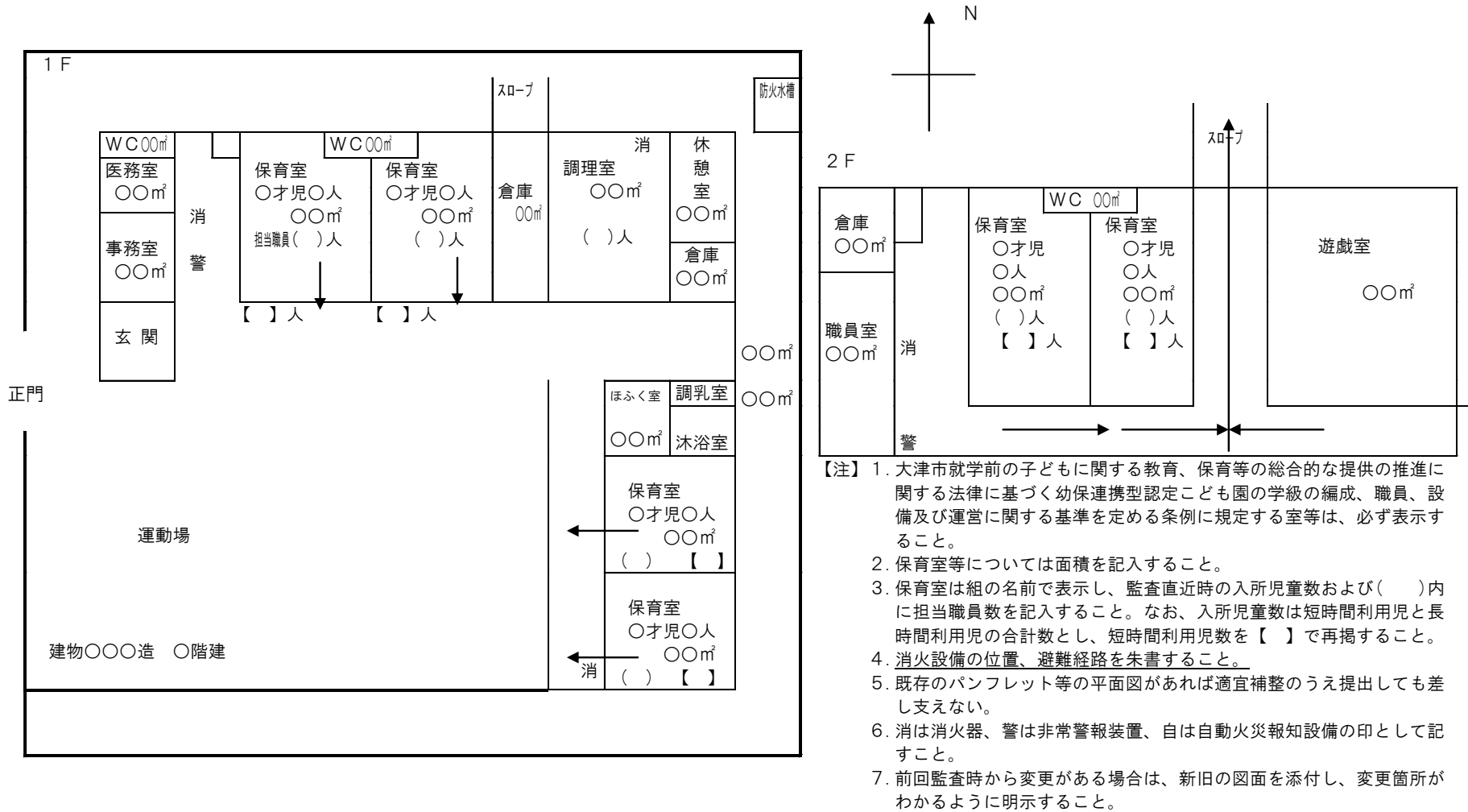
(5)施設平面図
