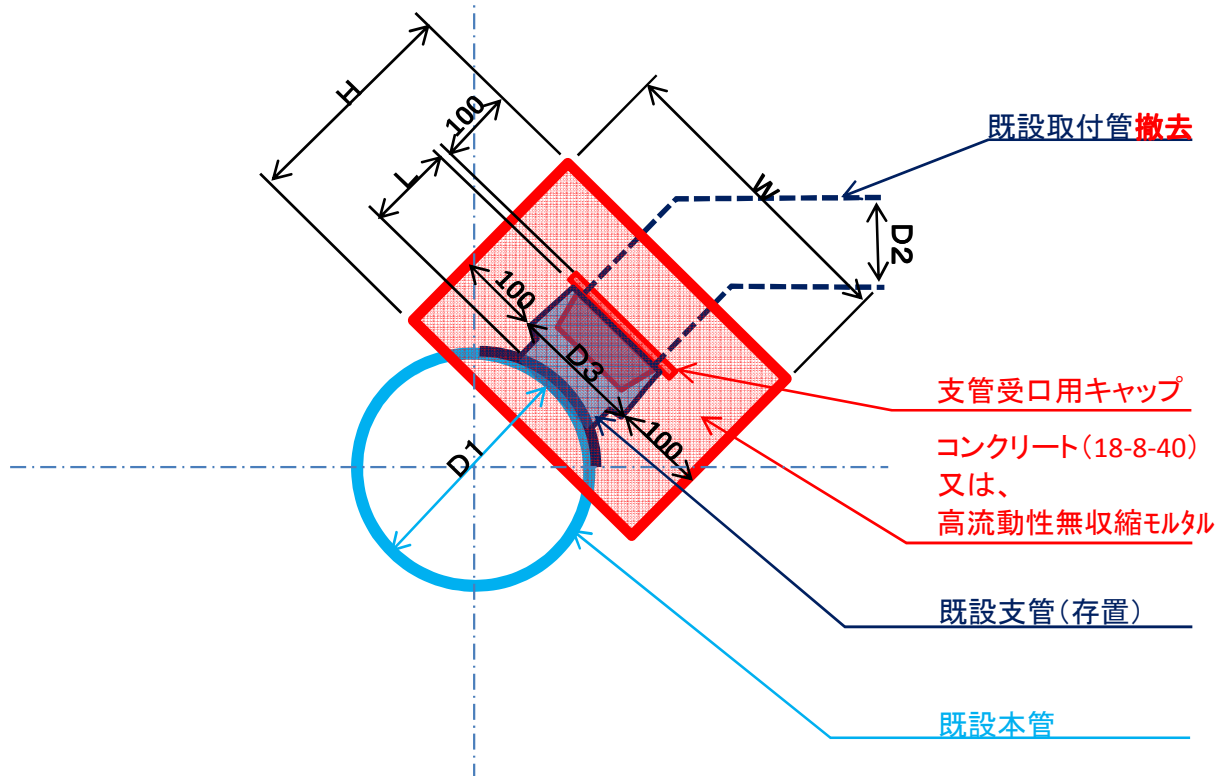
本管：硬質塩化ビニル管の場合
