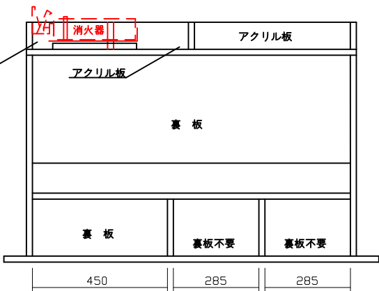
背面図
