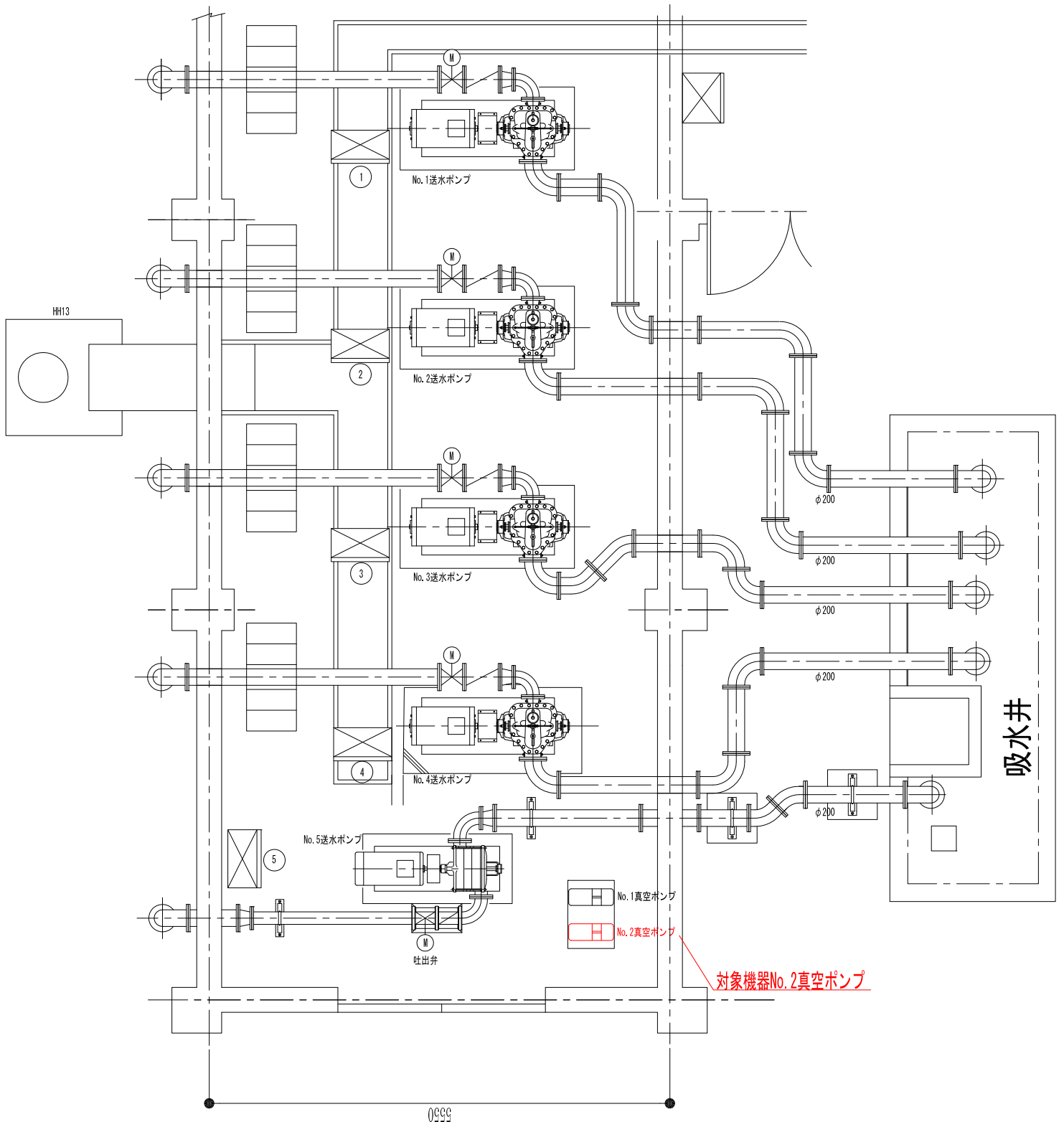
高区系送水ポンプ室平面図
