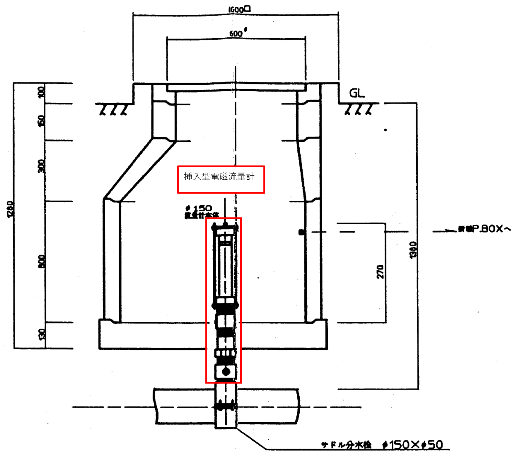
φ 150 挿入型電磁流量計詳細図
