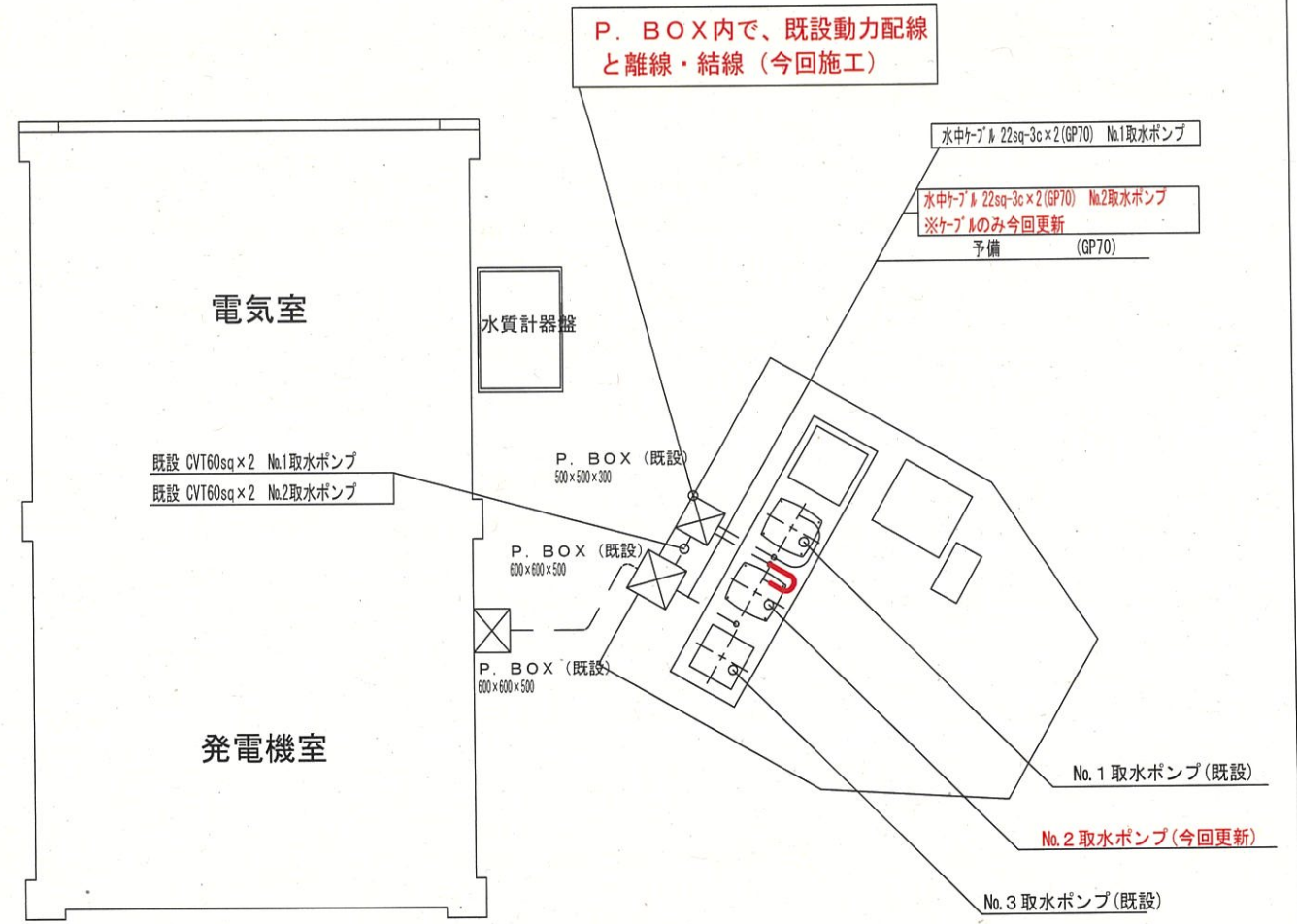
電気配線図 Non Scale
