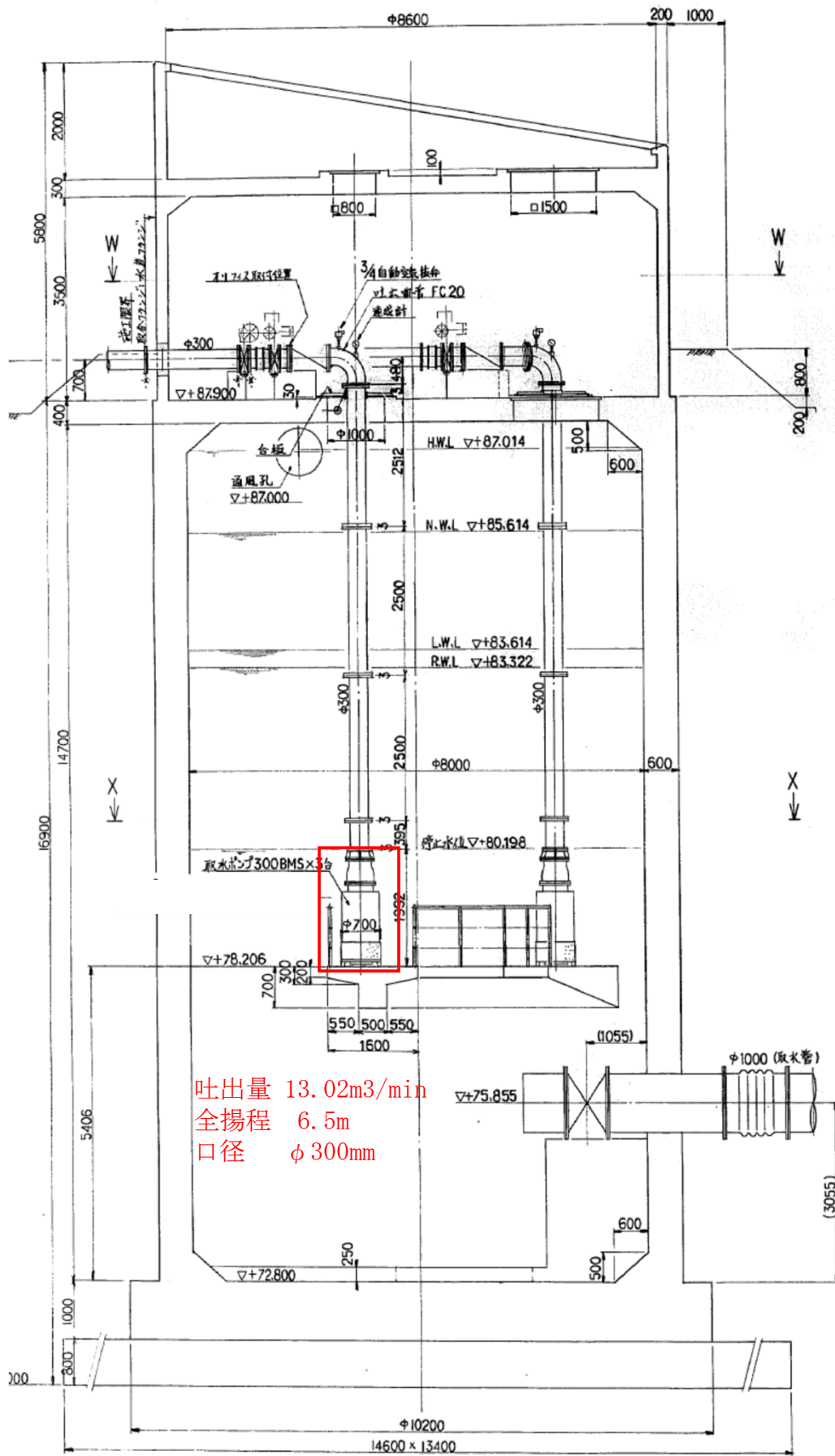
断面 VV
