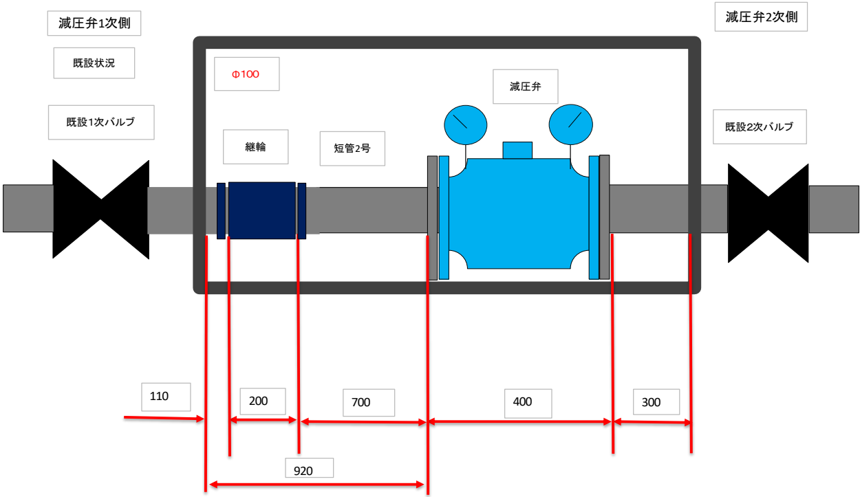
曾束減圧弁既設状況
