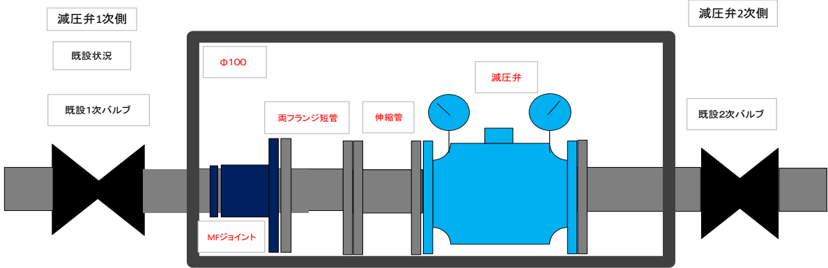
曾束減圧弁取替後状況
