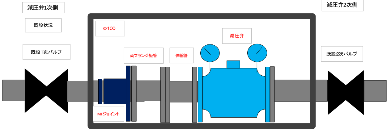
雄琴減圧弁取替後状況
