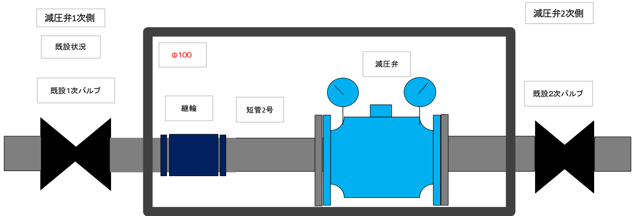
雄琴減圧弁既設状況
