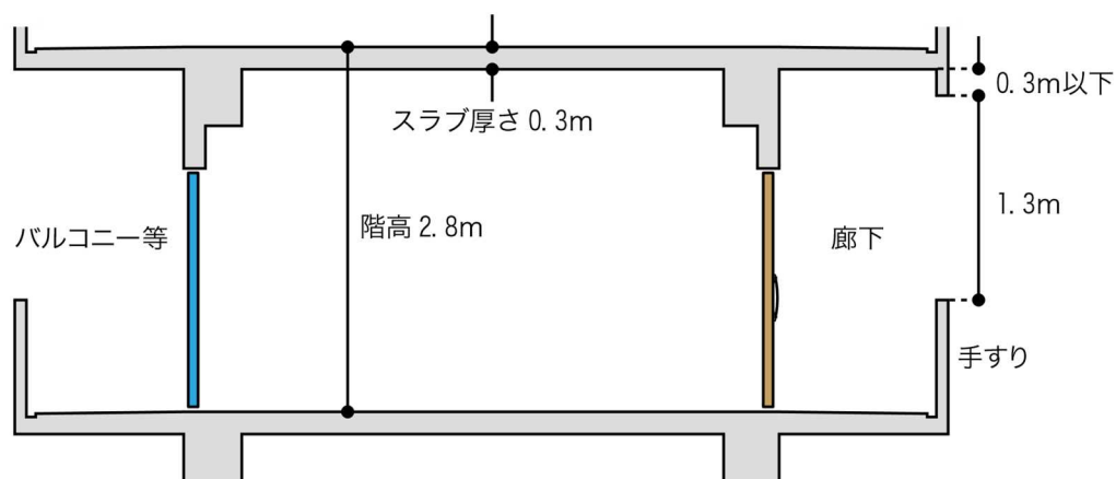
(断面図)
