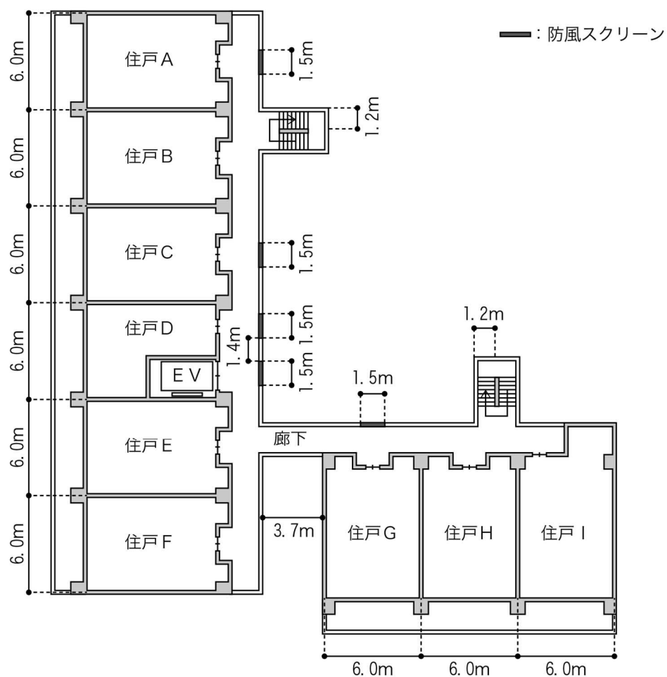
(平面図)
