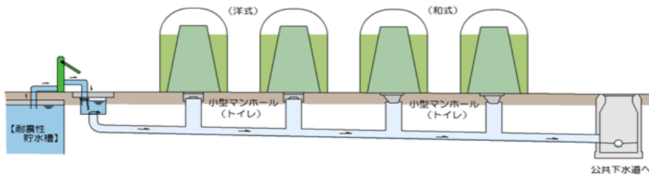
【マンホールトイレのイメージ図】
