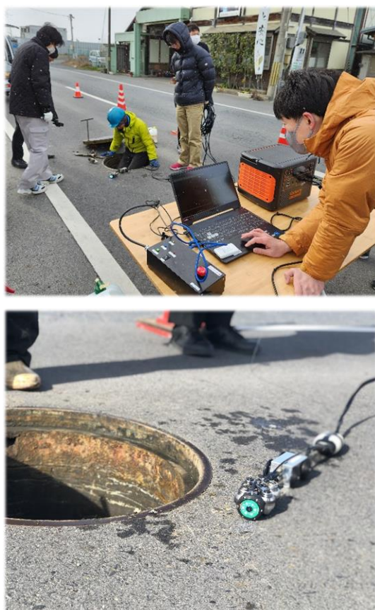
【小口径圧送管点検ロボット実証実験】
