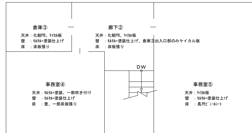
3階イメージ図（平面）
