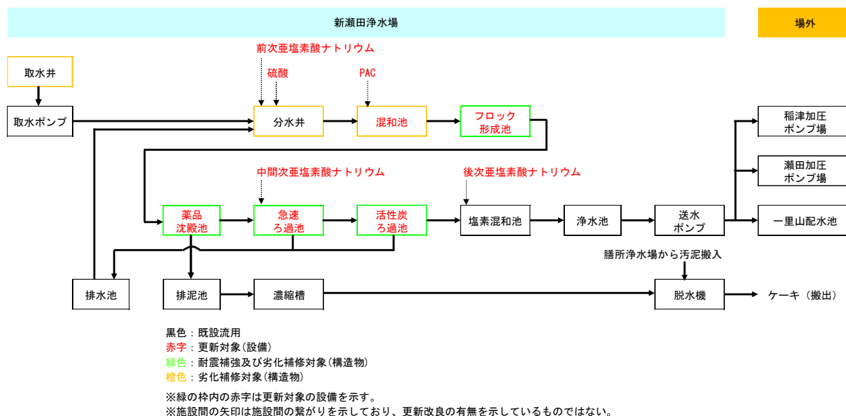
図－ 2 浄水フロー（新瀬田浄水場）
