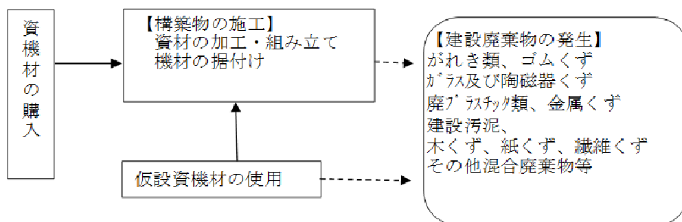
図－２ 構築物施工に伴う産業廃棄物の発生
