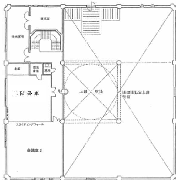
二階平面図
