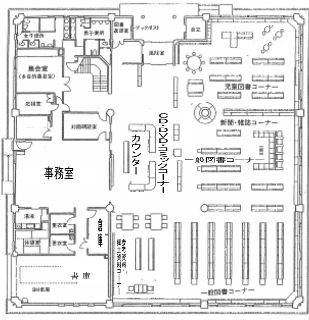
一階平面図
