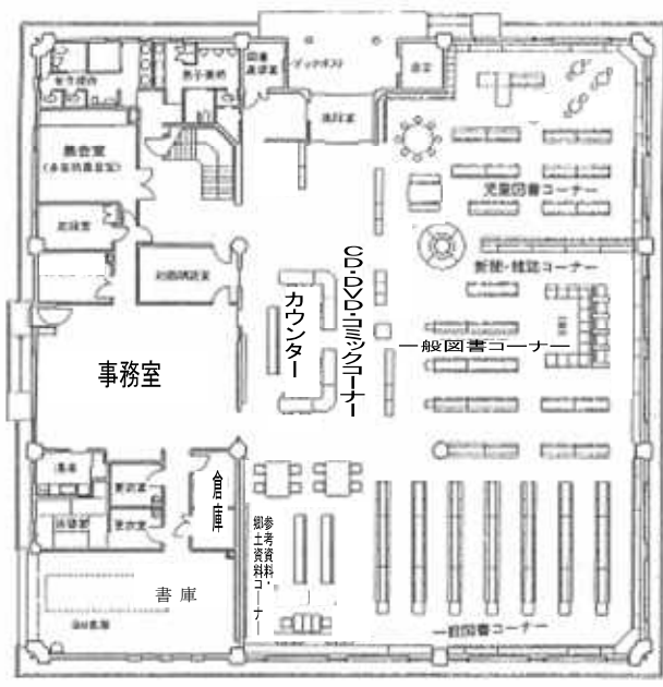
一階平面図
