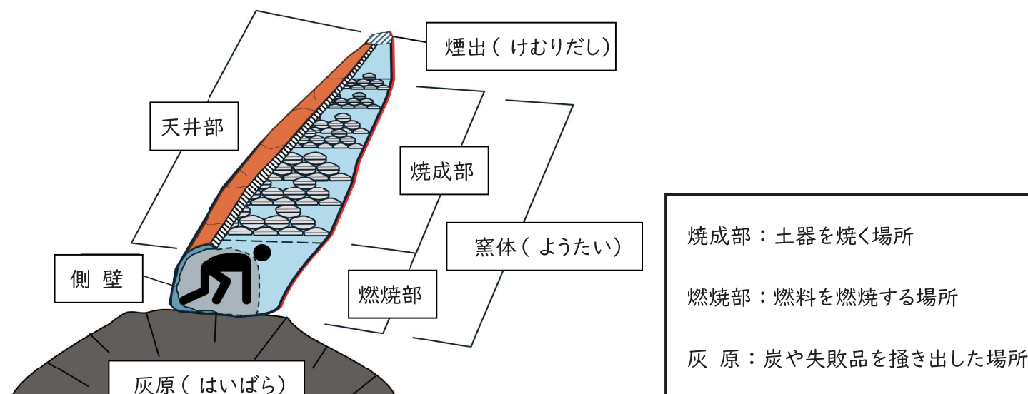
図2 須恵器窯の各部名称
