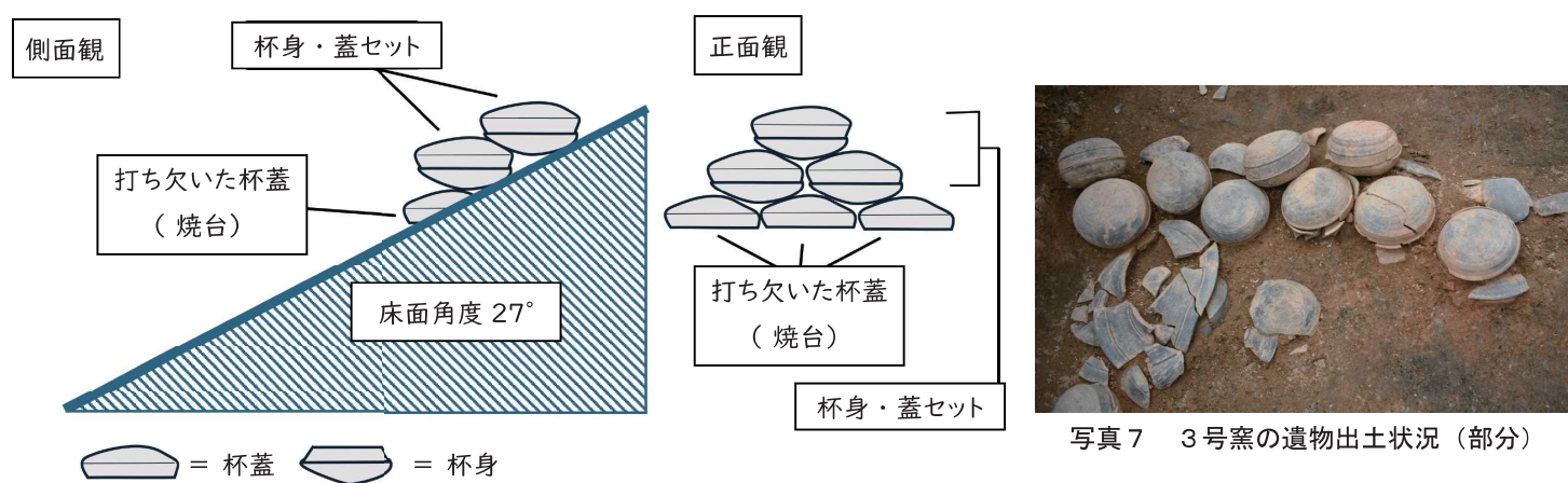
図4 3号窯窯詰模式図
